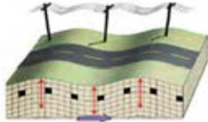
شکل ۴-۶: موج S
