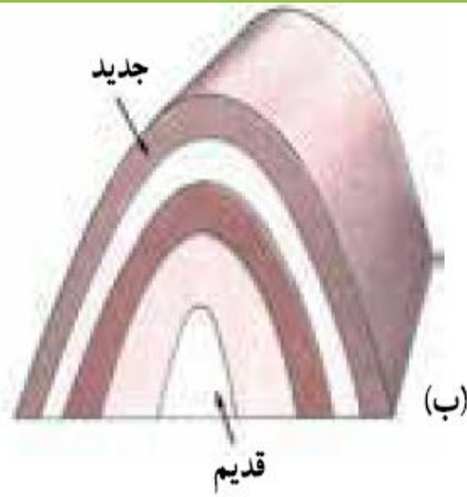
شکل ۳-۶- انواع چین
