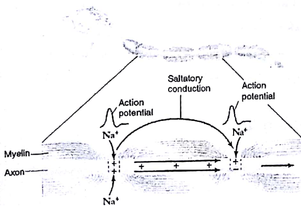
شکل ۸- هدایت جهشی در نوروں میلین دار
