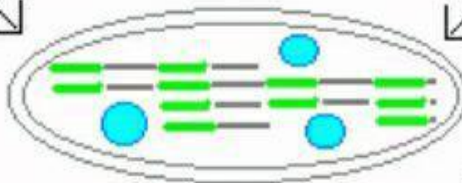
chloroplast
