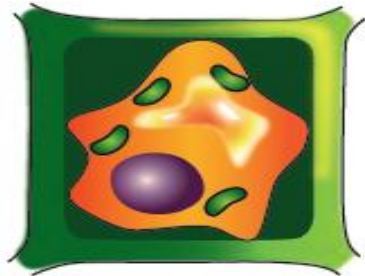
پلاسمولیز
